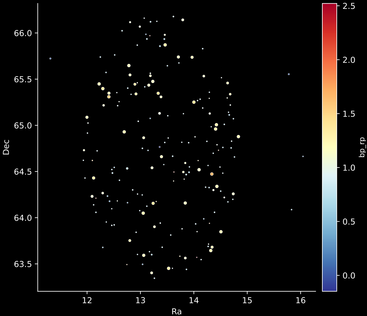
APOGEE DR17 Field: [CVZ_OB18_btx] Stars: 190
