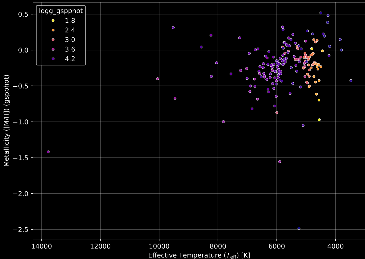
APOGEE DR17 Field: [CVZ_OB18_btx] Stellar Population Parameters (n= 190)
